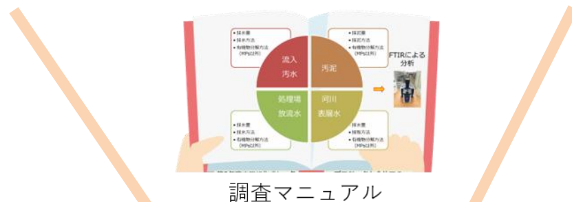
3-(3) 河川
